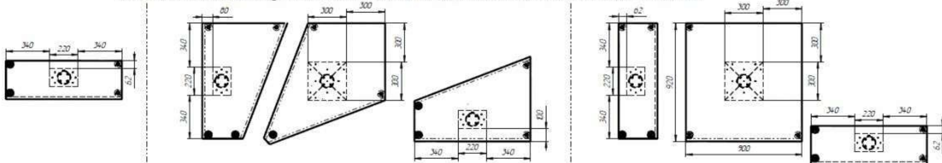
Разметка ступеней для засверливания под болта, болты крепления (отверстие \phi 9 мм) и стойки перил (отверстие \phi 26 мм)
